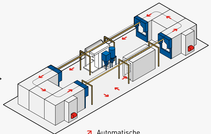
➔ Automatische Pulverbeschichtungsanlage
